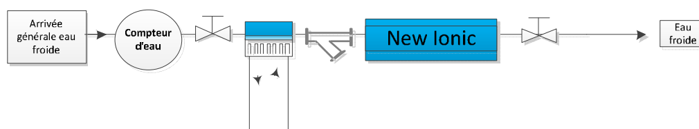
Schéma d'installation sur l'arrivée générale
