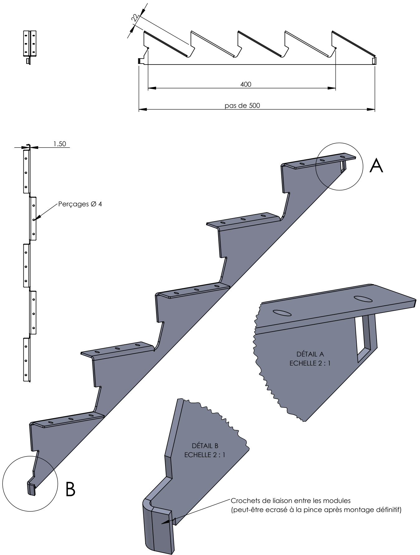
FORMAT FEUILLE A4 - éch: 1: 5 - pièce en acier inoxydable ép: 1. 5 mm - produit développé pour: www.matériaux-naturels.fr - reproduction interdite
