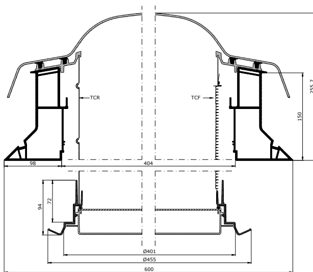
Vue en coupe (schématisée)
