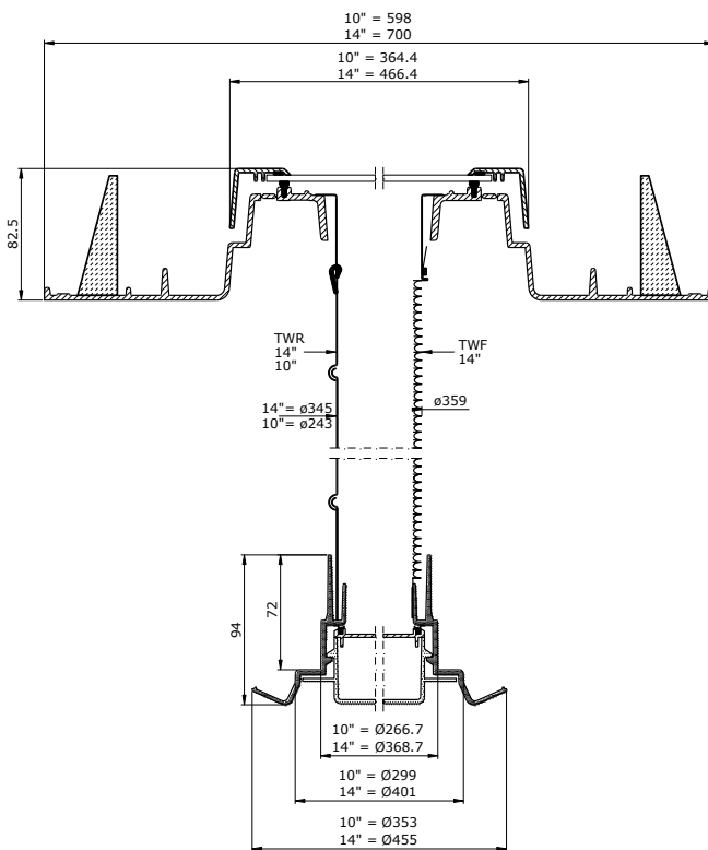
Vue en coupe schématisée
