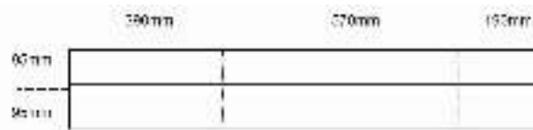
Figure 2-6 : Diffuseur métallique en aluminium vue de dessus
