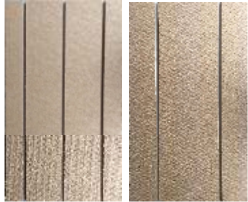
Figure 2-1 : Plaques de fibre de bois ECO+ en pas de 20 et 30cm
