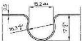
Figure 2-5 : Coupe diffuseur métallique en aluminium
