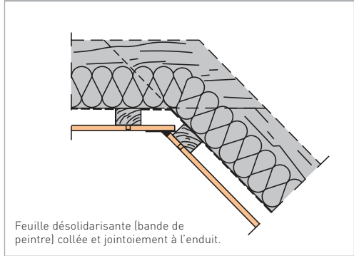
Figure 18 : 2. Jointolement avec feuille désolidarisante
